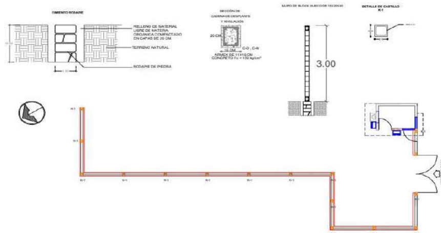
CASETA DE VIGILANCIA (OBRA NUEVA).
