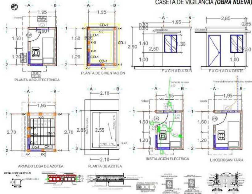
CASETA DE VIGILANCIA (OBRA NUEVA).
